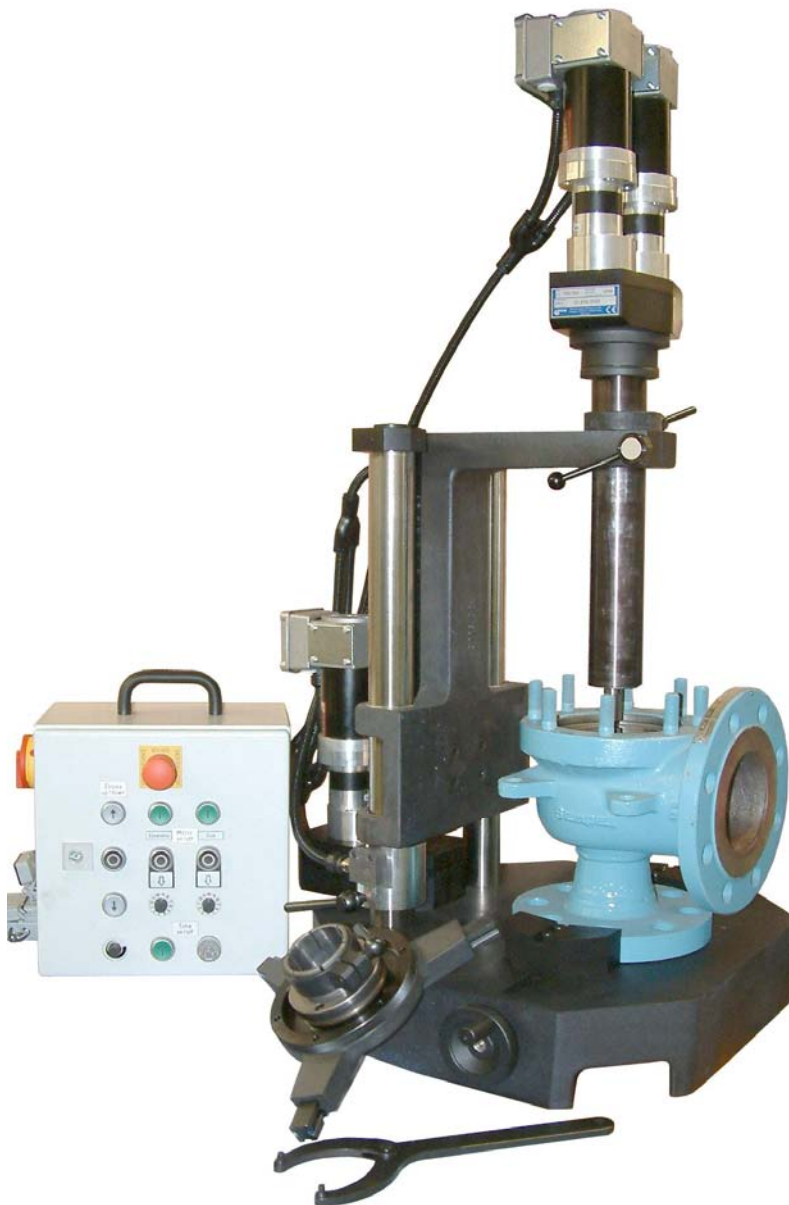
TSV-300 auf Ständer
